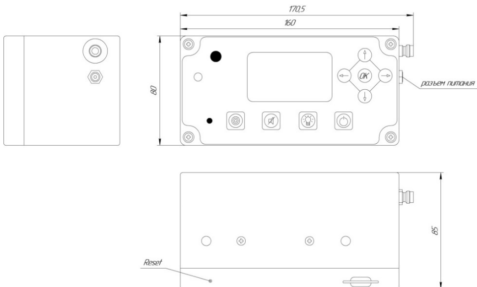
Рисунок 1. Габаритный чертёж прибора
